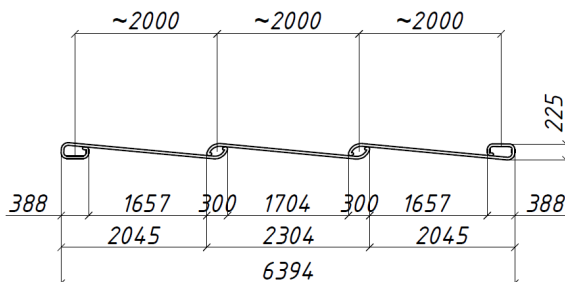
Крафтовий Паркан Хвиля
