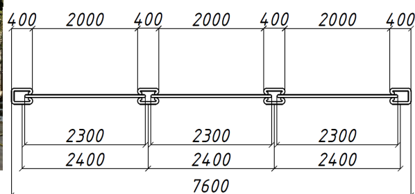
Крафтовий Паркан з маленьких колон (400 мм) та прямими панелями (2300 мм)
